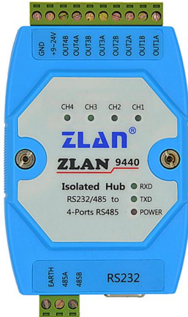
图 3 9440 接口图
