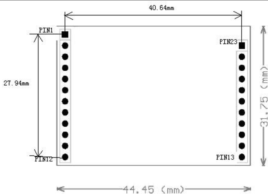
图 5 ZLSN2003B 正面引脚图
